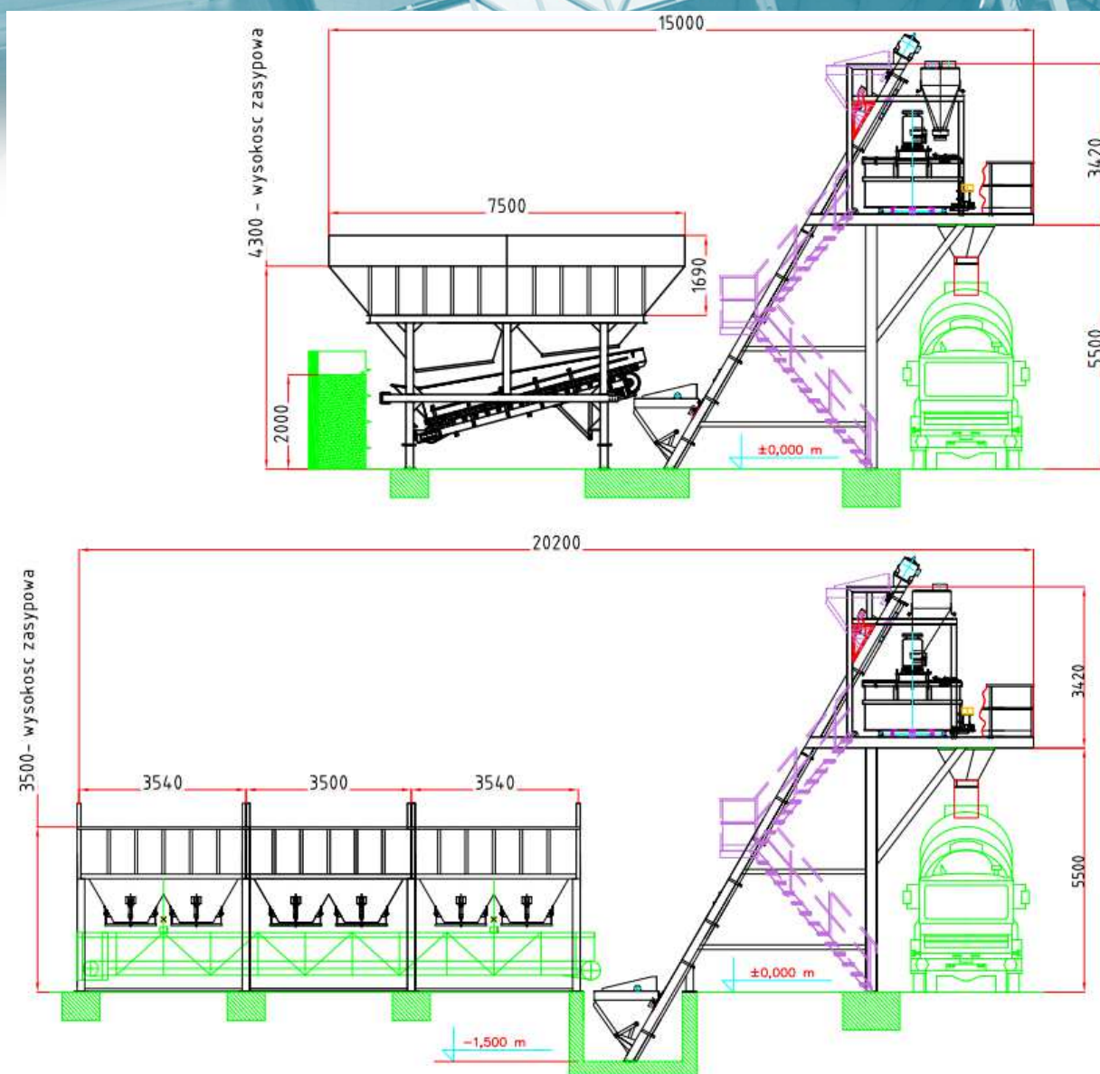
Węzeł betoniarski
